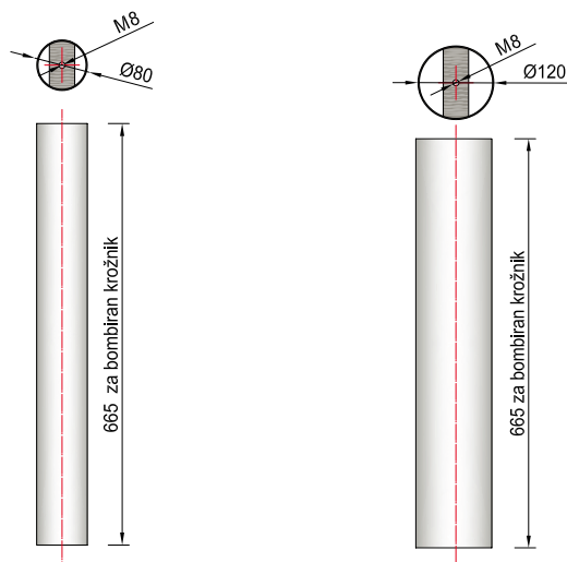
Pillar of table leg MAXIS, cambered / Säule MAXIS, bombiert
