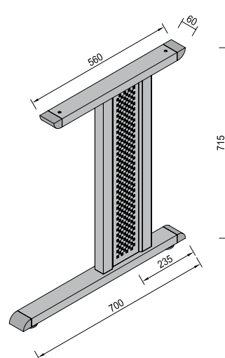
DOHA 700 mm, C-leg / T-Fuß
