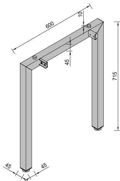
MILANO 600 mm, PLUS
