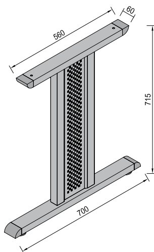
DOHA 700 mm, T-leg / T-Fuß
