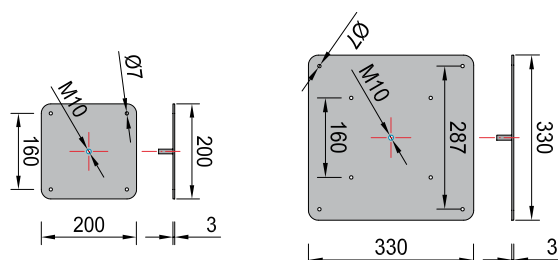
Support plate MAXIS, cambered / Tragplatte MAXIS, bombiert
