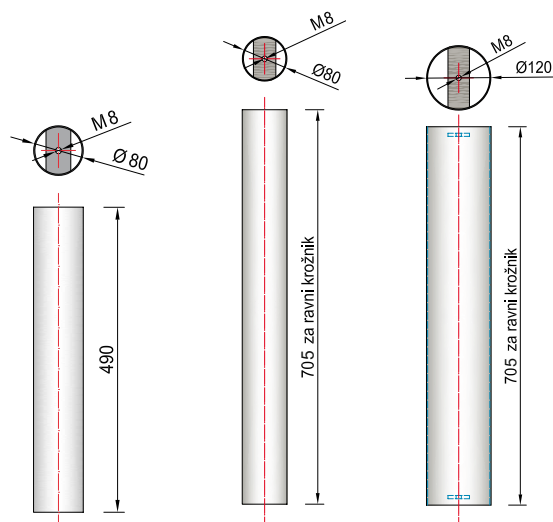
Pillar of table leg MAXIS / Säule MAXIS
