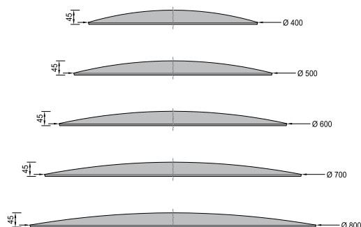
Plate MAXIS, cambered / Bodenplatte MAXIS, bombiert
